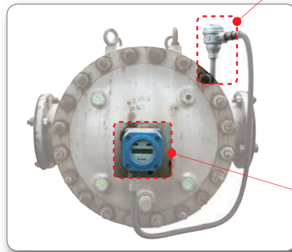
電子式自動温度補正装置付・ウルトラオーバル流量計
